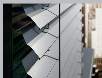
Profil Z90 - obrót lamel: 90° - max szer. 4500 mm - max pow. 16m 2
