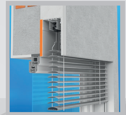
Żaluzja fasadowa Box S20 - do zabudowy z odsadzeniem na dodatkowe ocieplenie 20 mm
