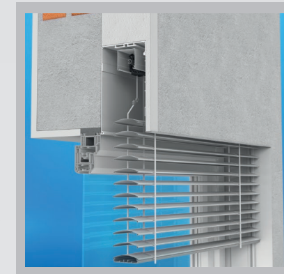
Żaluzja fasadowa Box - do zabudowy
